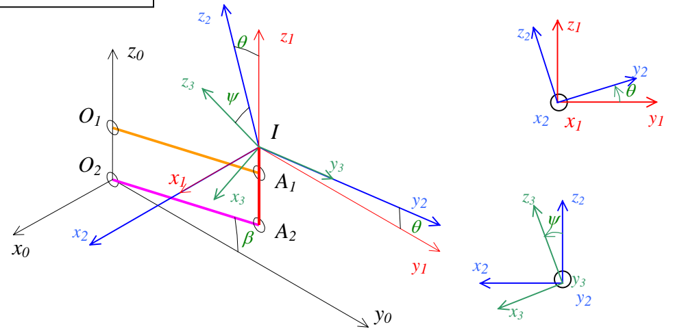
Figure 3 : Schéma cinématique du simulateur
