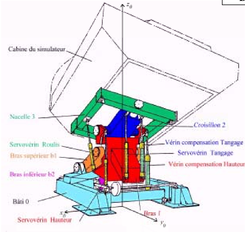
Figure 1 : Description du simulateur
