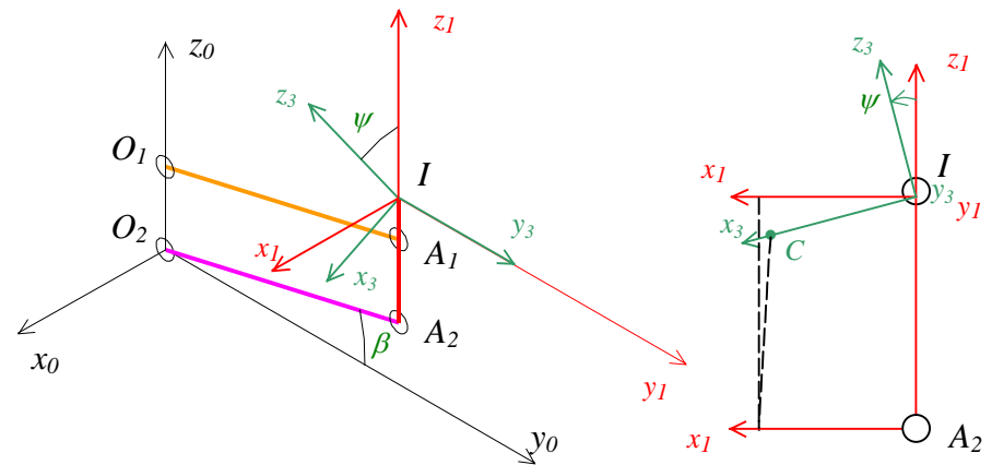
Figure 4 : Schéma cinématique du simulateur dans le cas d'un tangage nul
