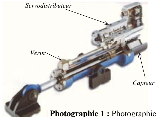
Figure 1 : Description du simulateur
